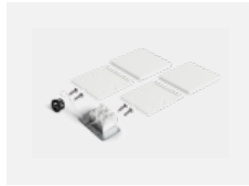
00-20100, B 2xEndcappe - Metall, Klemmleiste 3-polig, Kabeldurchführung; Lipo80/Lina80
